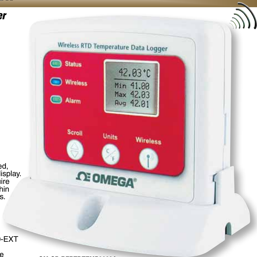
OM-CP-RFRTDTEMP2000A shown actual size.
