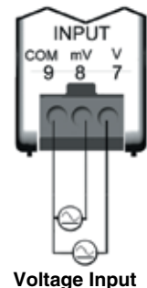
Voltage Input
