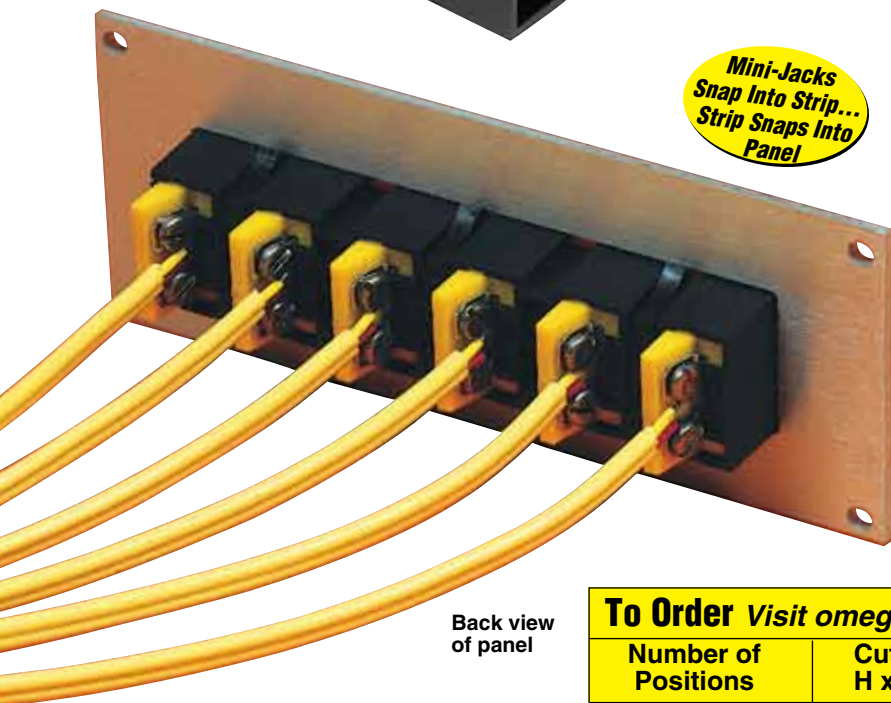
MSS-06 shown
